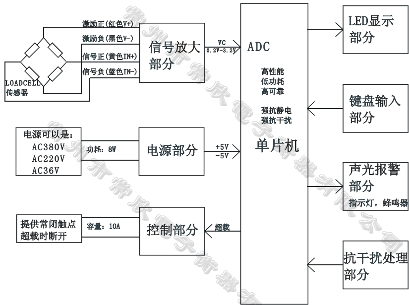
电气原理示意图
