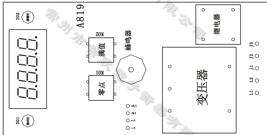
元件布置图
