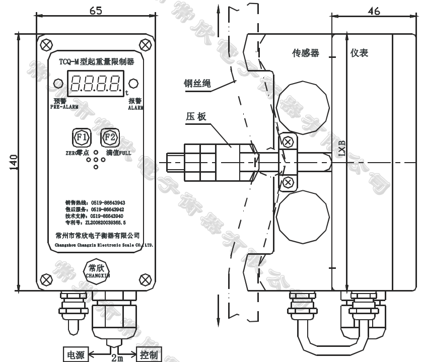
总体连接图
